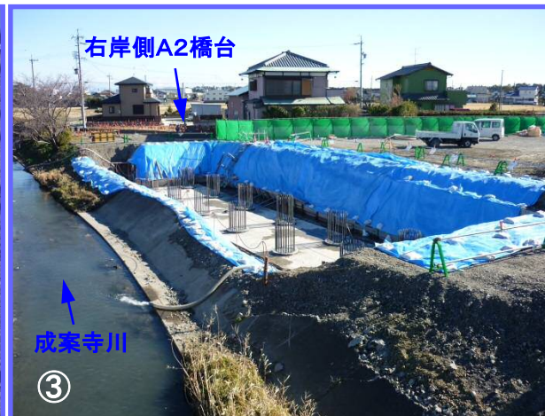
成案寺川に架かる新設橋梁工事のうち、右岸側では杭基礎工事が完了しました。年明けから鉄筋を組み始め、コンクリートを打設します。
