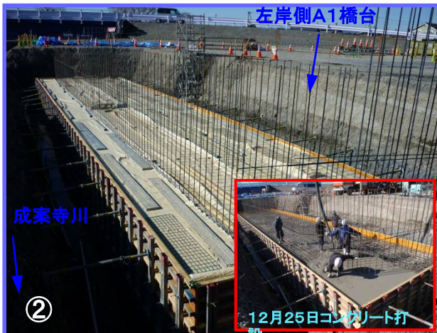
成案寺川に架かる新設橋梁工事のうち、左岸側では橋台下部のコンクリート打設が完了しました。年明けから橋台上部の作業に入っていきます。
